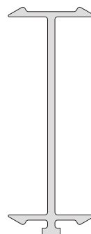
3010/ 13 Unión 257 g/m 24 barras de 6.150 mm.
