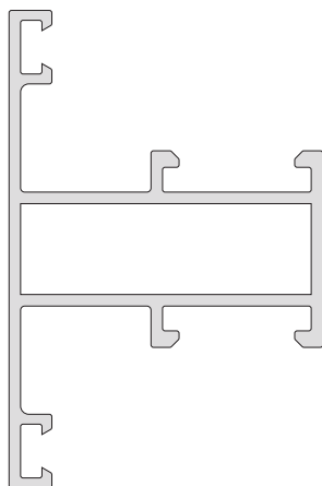
3010/ 64 Travesaño p/paño fijo curvo 720 g/m 6 barras de 6.150 mm.
