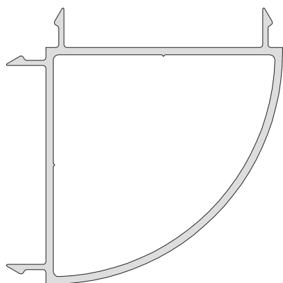
3010/ 62 Acople 90° 681 g/m 2 barras de 6.150 mm.
