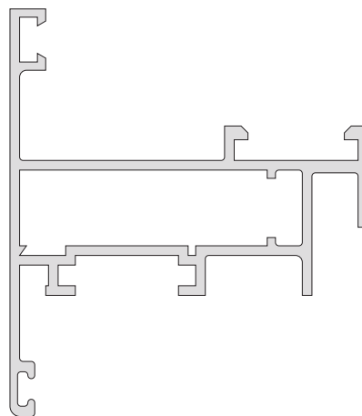
3010/ 27 Hoja ventiluz 864 g/m 6 barras de 6.150 mm.
